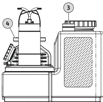
Fig. 6: Ontluchtingsaansluiting verzamelreservoir
