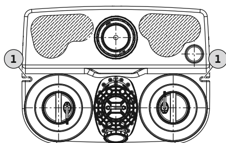
Fig. 2: Boven aanzicht opvoerinstallatie
