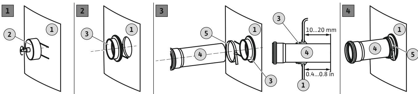
Fig. 5: Tulovirtauksen liittäminen
