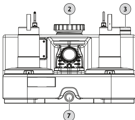
Fig. 7: Käsikäyttöisen kalvopumpun liitäntä
