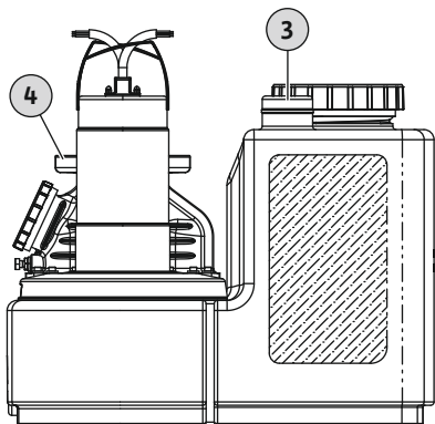
Fig. 6: Keräyssäiliön ilmanpoistoliitäntä
