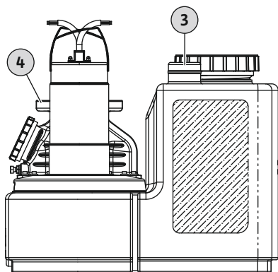
Fig. 6: Conexión de purga del depósito colector
