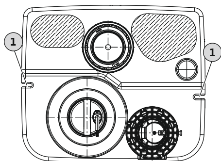
Fig. 2: Vedere de sus a modulului de pompare
