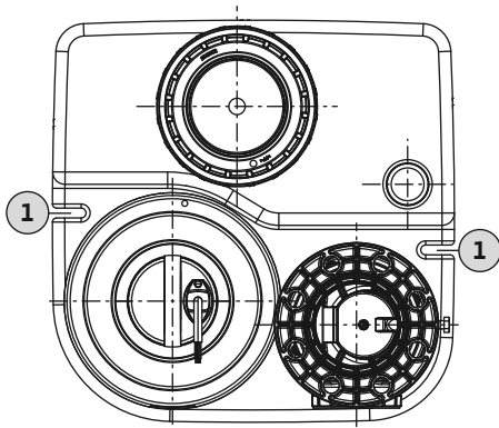
Fig. 2: Heveanlegg ovenfra
