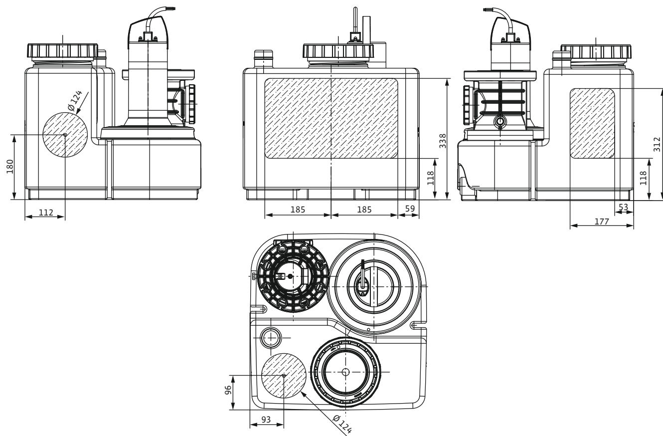
Fig. 4: Oblasti přítoku
