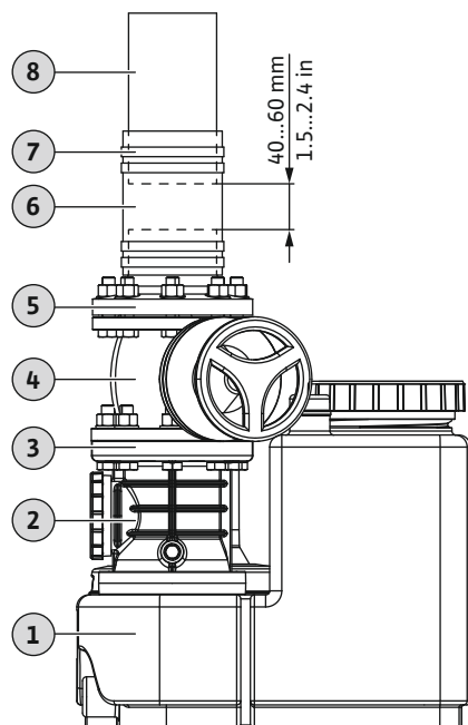
Fig. 3: Свързване на връзката за продухване
