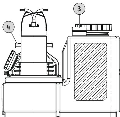
Fig. 6: Σύνδεση εξαερισμού δεξαμενής συλλογής λυμάτων
