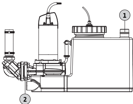
Fig. 8: Σύνδεση εξαερισμού δεξαμενής συλλογής λυμάτων
