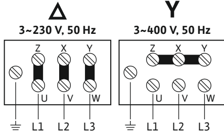
Fig. 4: Motor bağlantısı
