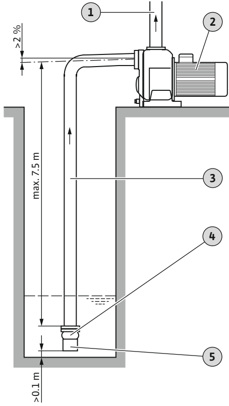
Fig. 3: Sabit kuru kurulum
