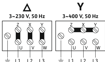
Fig. 4: Pripojenie motora
