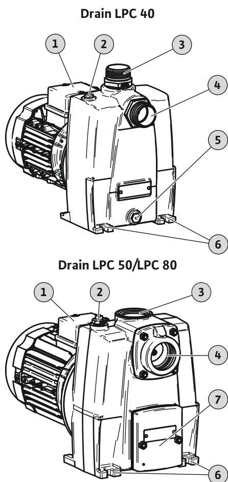
Fig. 2: Prehľad výrobku
