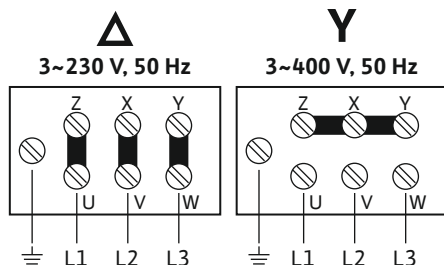
Fig. 4: Motorcsatlakozás
