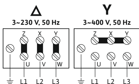
Fig. 4: Σύνδεση κινητήρα
