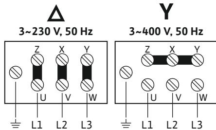
Fig. 4: Motoranschluss
