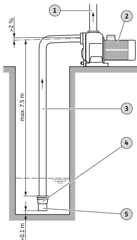
Fig. 3: Stationäre Trockenaufstellung
