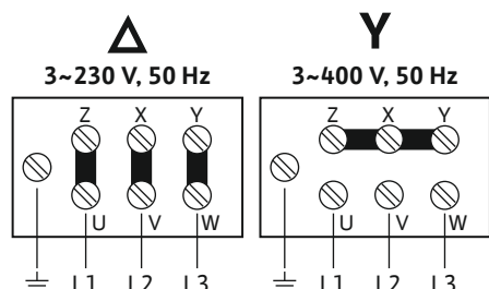
Fig. 4: Zapojení motoru
