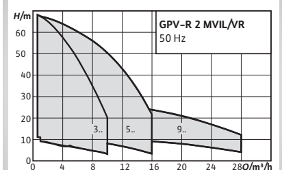
Curve di preselezione
