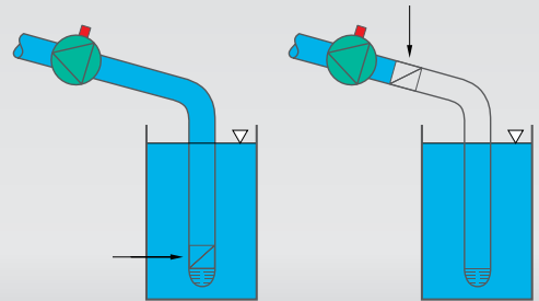
Монтаж з використанням приймального або зворотнього клапанів
