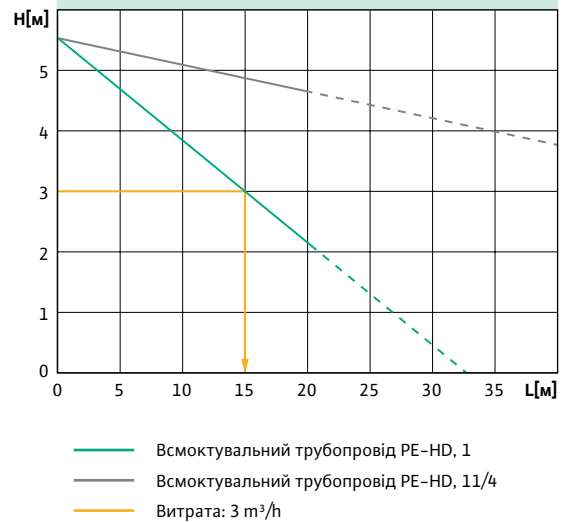
Залежність між довжиною всмоктувального трубопроводу та висотою всмоктування
