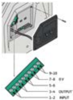
Електронна розширювальна плата
