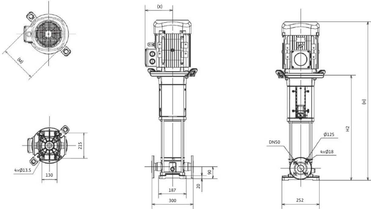
외형치수 및 중량, 전기자료 (60Hz, 2극)
