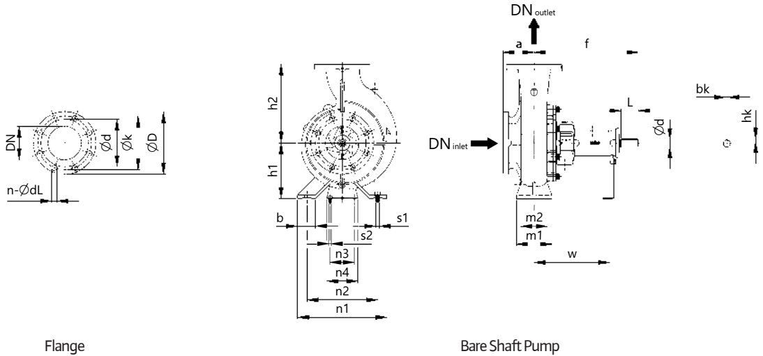
Flange
