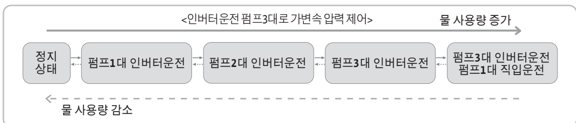
Combi type 운전 Logic(3-인버터, 4-펌프 시스템 기준)
