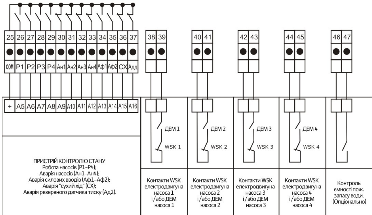
Мал.4а - Зовнішні сигнальні та контрольні ланцюги.
