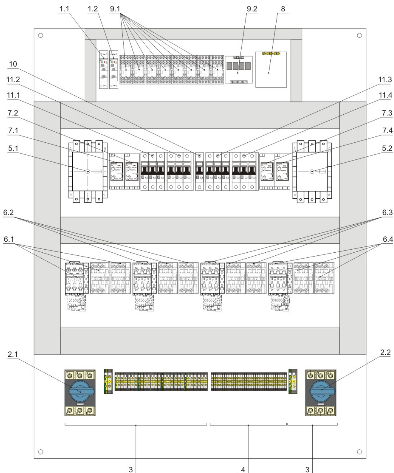
Мал.26 - Внутрішній вигляд
