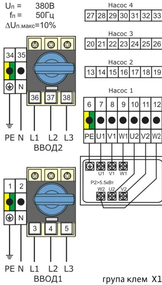
Мал.3 - Силові ланцюги для 2 - 4х насосних стацій
