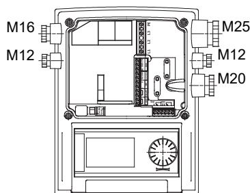
Fig. 29: Kabelio priveržikliai
