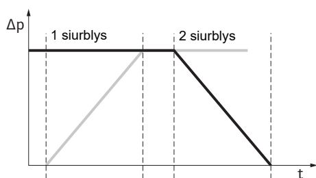
Fig. 11: Siurblių apsikeitimas, schema
