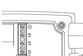
Fig. 27: Elektros gnybtai
