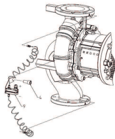
Lent. 14: Diferencinio slėgio jutiklio prijungimas
