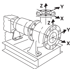
Fig. 22: Apkrovos variantas 1A
