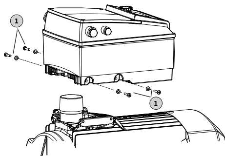
Fig. 49: Elektronikos modulio ryšys – variklis
