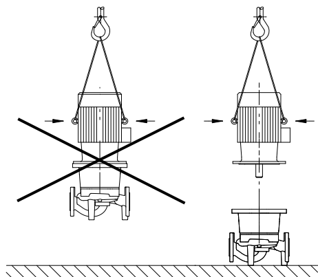
Fig. 2: Variklio transportavimas
