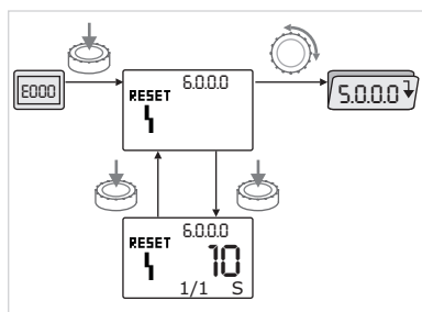
Fig. 50: Klaidų atvejų navigacija
