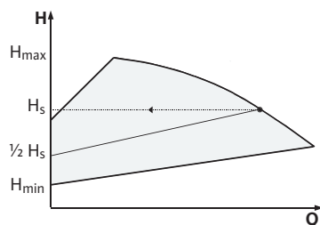
Fig. 7: Reguliavimo režimas \Delta p -v
