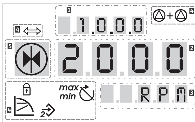
Fig. 36: Ekranų struktūra
