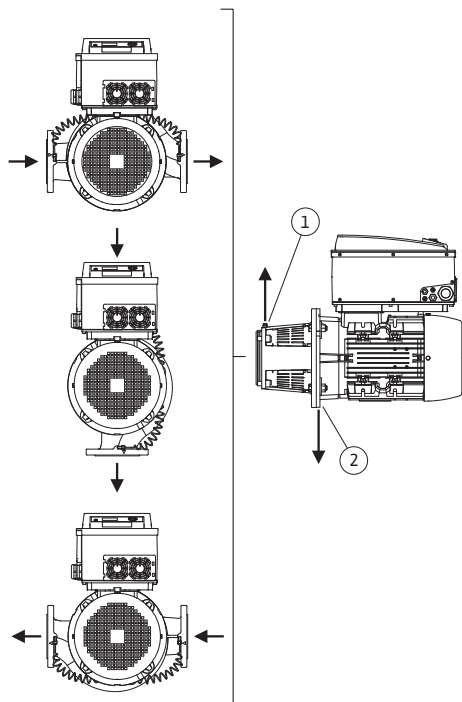
Fig. 14: Leistinos montavimo padėtys su horizontaliu variklio vėliu
