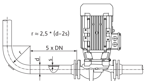
Fig. 18: Išlyginimo linija prieš siurbį ir už jo
