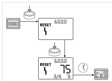
Fig. 55: B tipo klaidos patvirtinimas (X &lt; Y)
