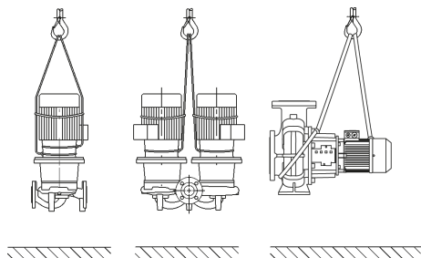
Fig. 1: Siurblio transportavimas
