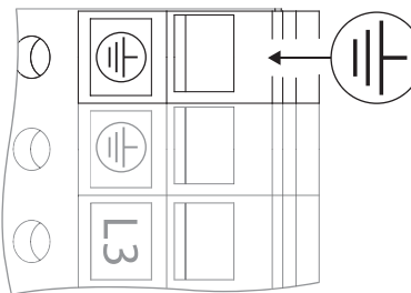
Fig. 28: Papildomas įžeminimas, variklio galiai esant nuo 11 kW
