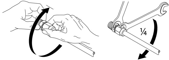
Fig. 19: Dar pasukite suveržimo žiedo varžtą per 1/4 pasukimo
