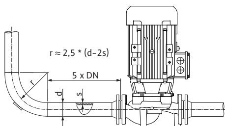
Fig. 18: Išlyginimo linija prieš siurblį ir už jo
