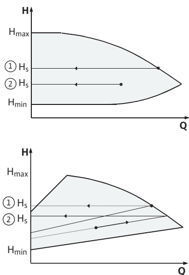
Fig. 32: Reguliavimas \Delta p-c/\Delta p-v
