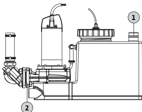
Fig. 6: Surinkimo rezervuaro nuorinimo jungtis
