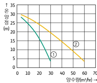
성능곡선도
