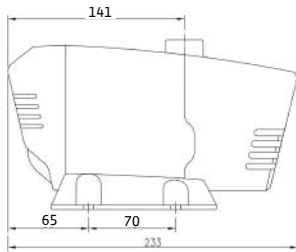
외형치수
