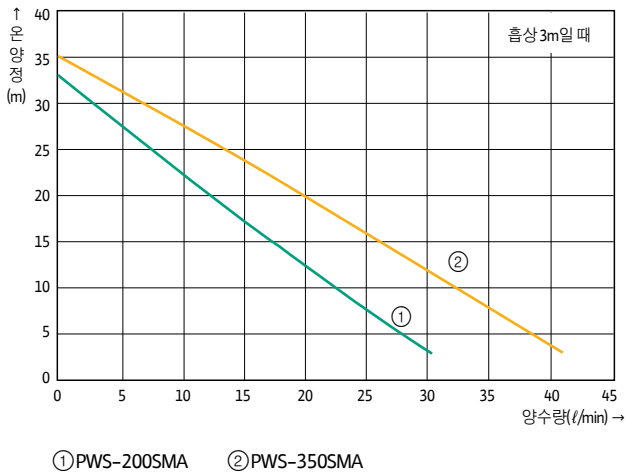
성능곡선도
