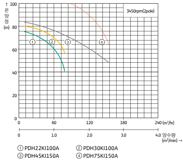
성능곡선도
