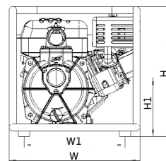
외형치수
