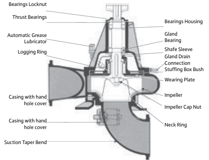
수직형 오수펌프
