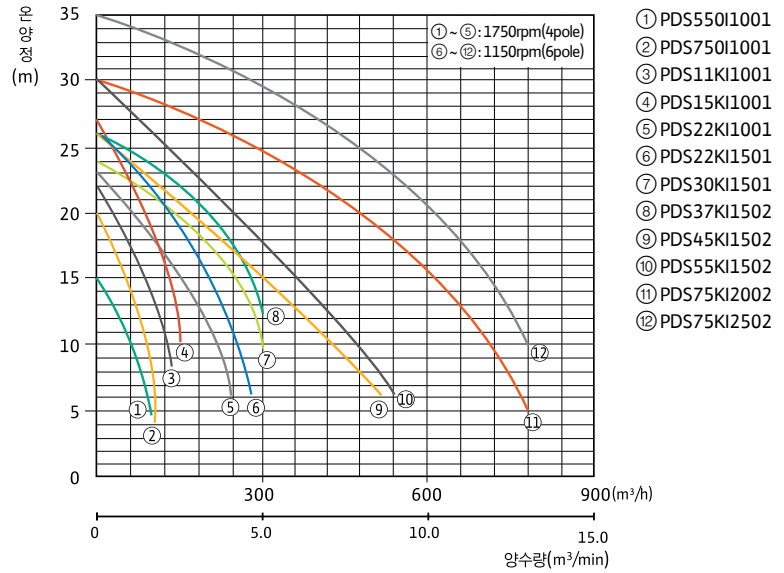
성능곡선도
