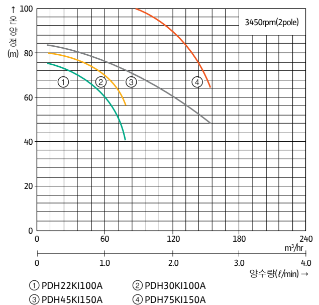
성능곡선도
