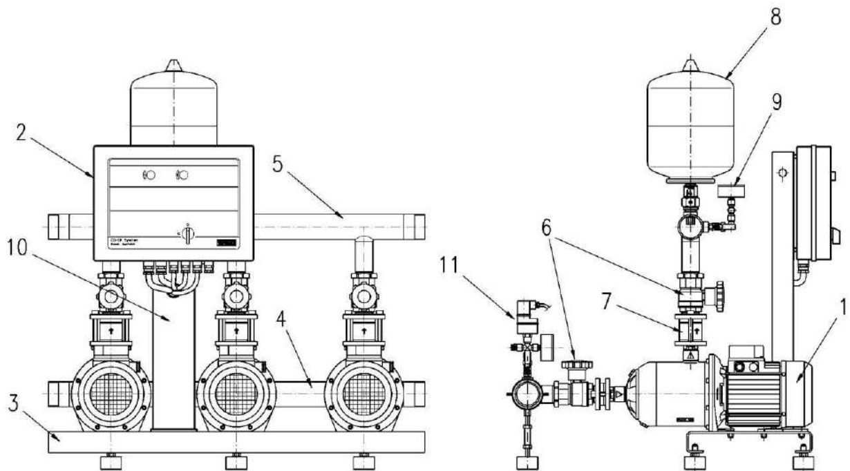
Малюнок 1. Установка з насосами МНІ та приладом керування ER
