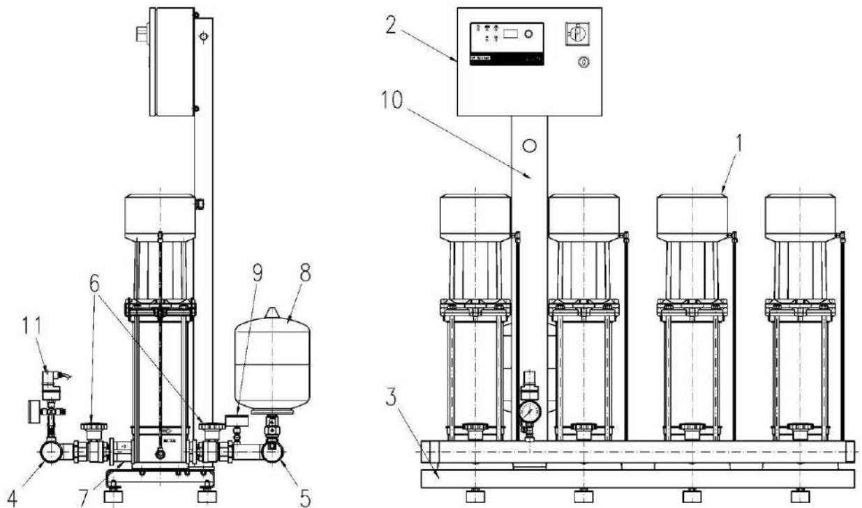
Малюнок 1. Установка з насосами МНІ та приладом керування ER
