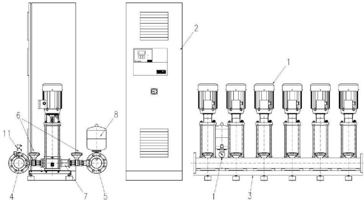
Малюнок 3. Установка з насосами MVI та приладом керування CR в окремо стоячій шафі
