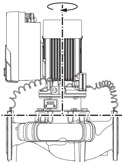
Fig. 10: Leistinos montavimo padėtys su vertikaliu variklio vėlu
