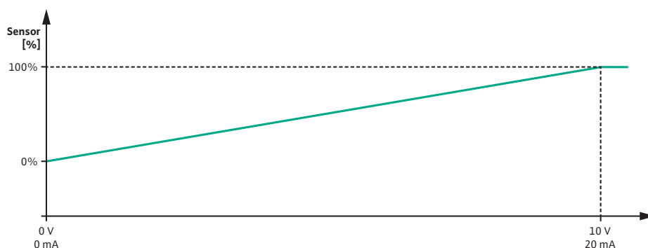
Fig. 75: Analoginio įeigos signalo AI1 veikimas: Signalų tipo jutiklio vertė 0 ... 10 V / 0 ... 20 mA
