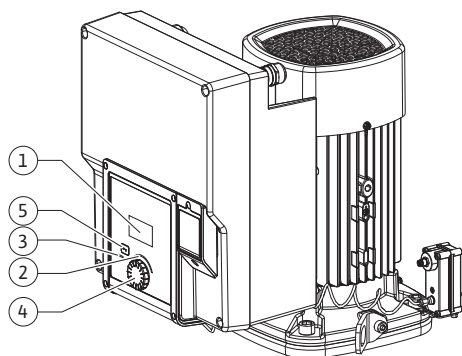
Fig. 27: Valdymo elementai
