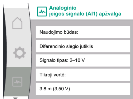
Fig. 95: Analoginio įėjus signalo (AI1) apžvalga
