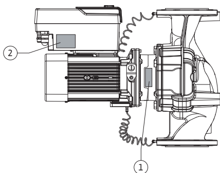
Fig. 2: Vardinės kortelės
