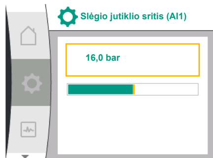
Fig. 71: Slėgio jutiklio diapazono nustatymas
