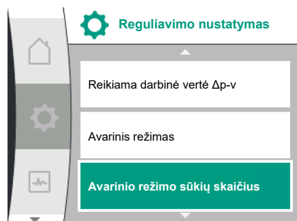
Fig. 44: Avarinio režimo sūkių skaičiaus nustatymas
