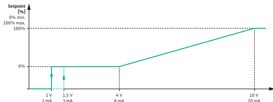
Fig. 79: Analoginio signalo AI2 veikimas: Signalų tipo 0 ... 10 V / 0 ... 20 mA reikiama darbinė vertė
