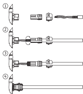
Fig. 25: Gnybtų ekranavimas
