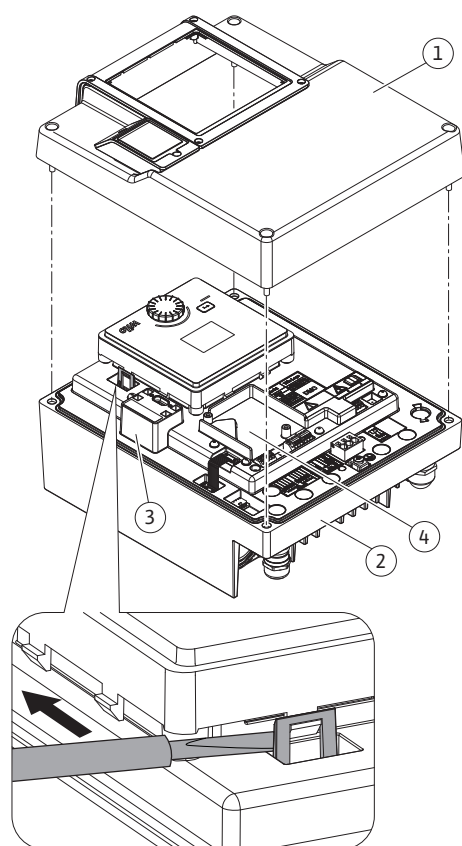
Fig. 26: Elektronikos modulis
