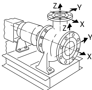
Рис. 11. Допустимые усилия и моменты на фланцах насосов — насос из серого чугуна
