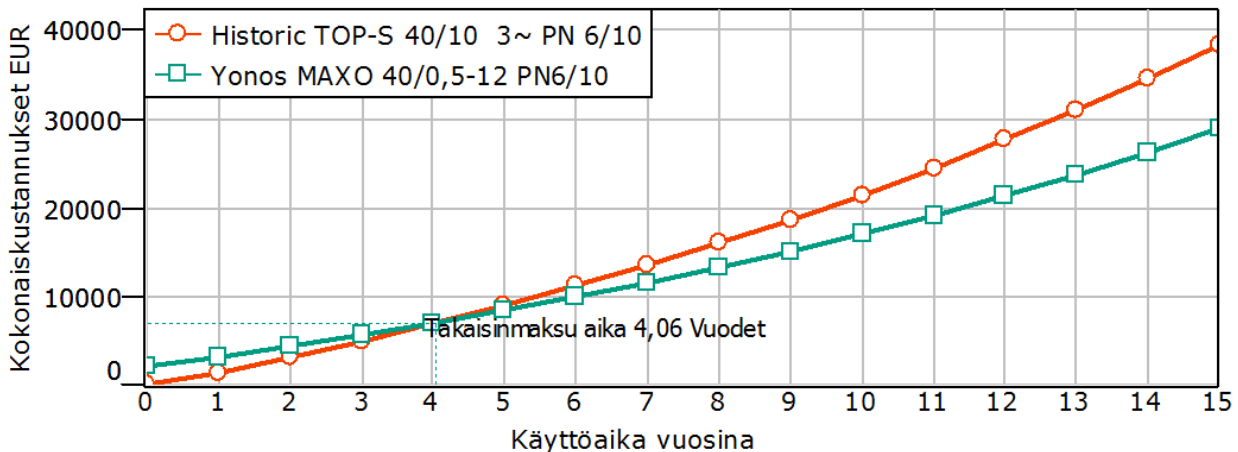
Taloudellisuusnäkökohdat - kustannuskäyrä
