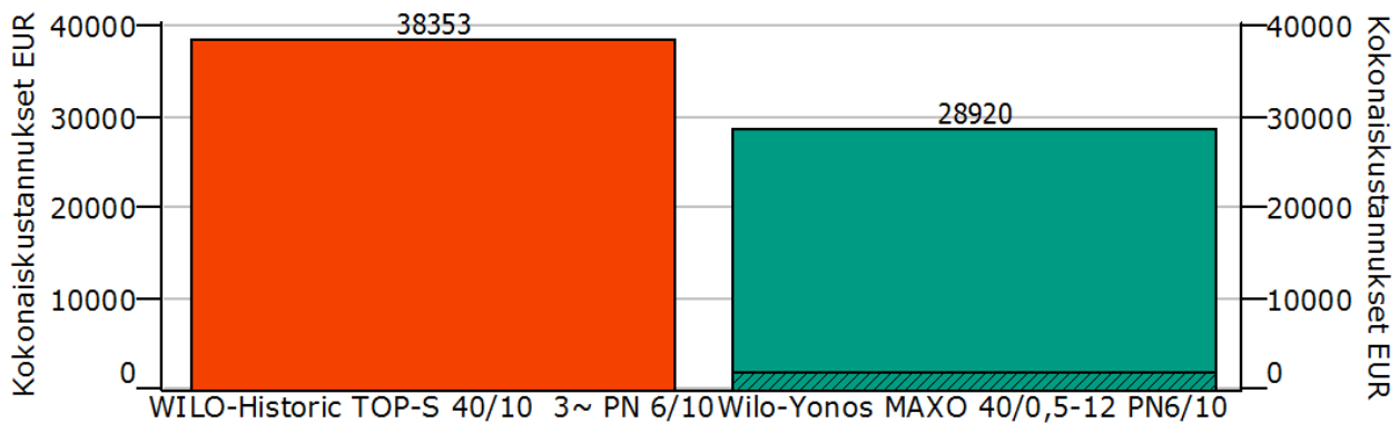
Taloudellisuusnäkökohdat 15 vuodeksi
