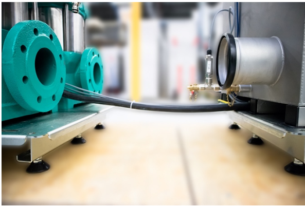
Kabelstrang zwischen Anlagenteilen.
