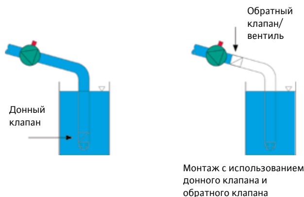
Монтаж всасывающего трубопровода
