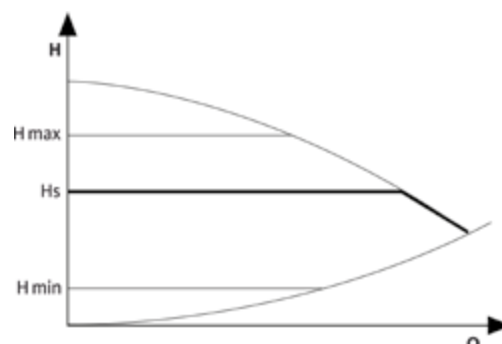
Способ регулирования \Delta p-c
