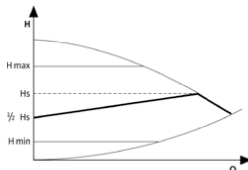
Способ регулирования \Delta p-v
