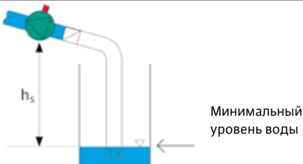
Высота всаса h_s
