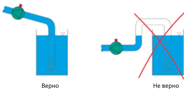
Монтаж всасывающего трубопровода
