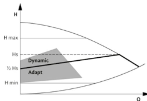
Способ регулирования \Delta p-v с Dynamic Adapt
