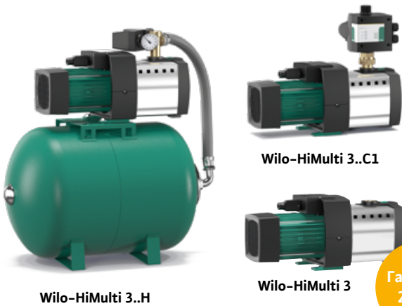
Wilo-HiMulti 3..H
