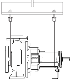
Fig. 3: Строповка насоса
