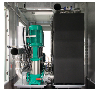
Innenansichten mit integrierter Trinkwasser-Trennstation.
