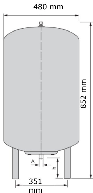
Réf. 2515525 – Vase d'expansion DE100
