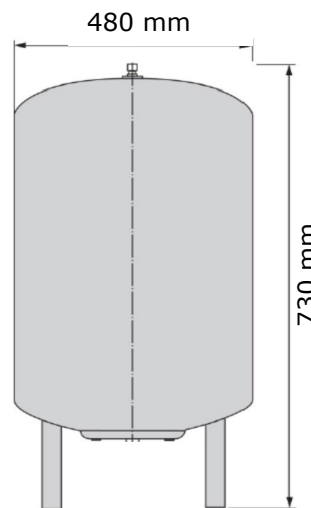
Expansievat DE 80
