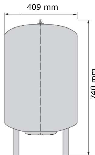
Expansievat DE 60
