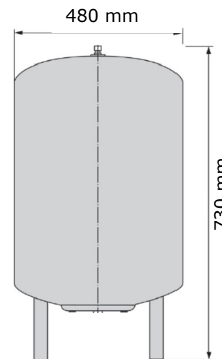
Expansievat DE 80
