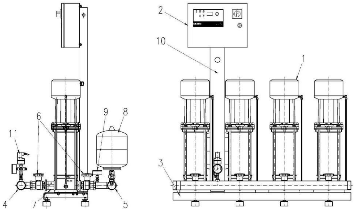
Малюнок 1. Установка з насосами МНІ та приладом керування ER
