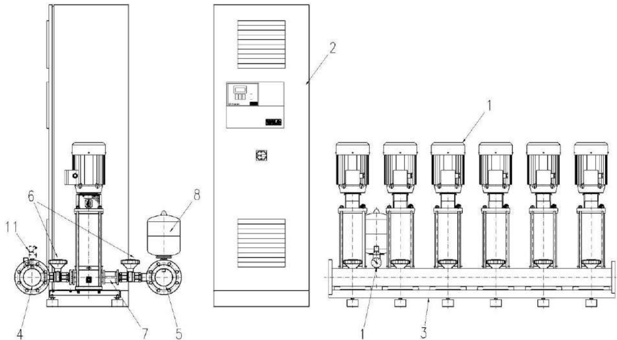
Малюнок 3. Установа з насосами MVI та приладом керування CR в окремо стоячій шафі
