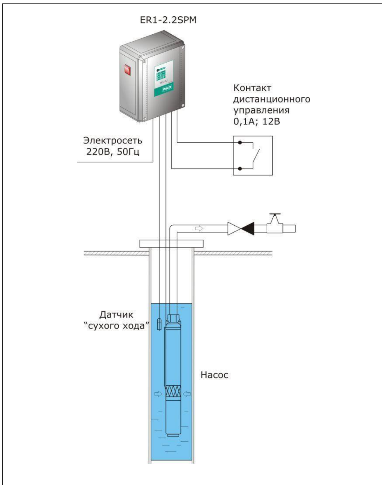
Рис.2 - Керування свердловинним (занурювальним) насосом
