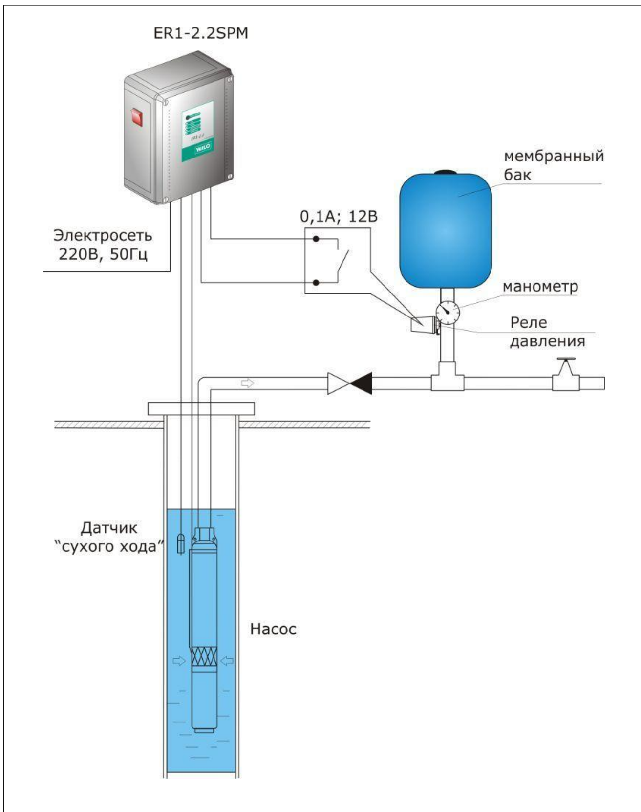
Рис.3 – Керування свердловинним (занурювальним) насосом в системі підвищення тиску
