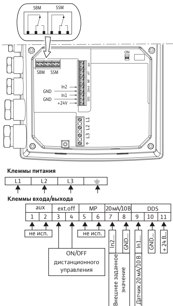
Схема подключения. 3–400 В ≤ 7,5 кВт
