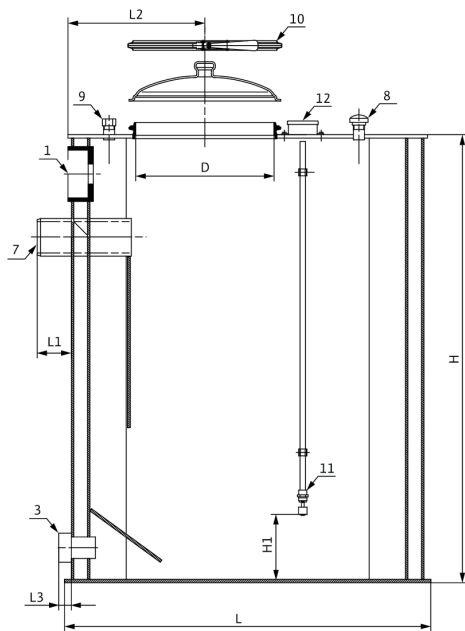
Габаритный чертеж 150 – 500 л, прямоугольный
