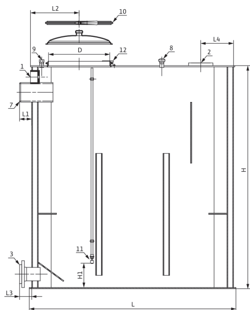
Габаритный чертеж 1500 – 3000 л, прямоугольный
