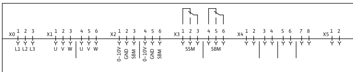
Схема подключения Smart Controller SCe
