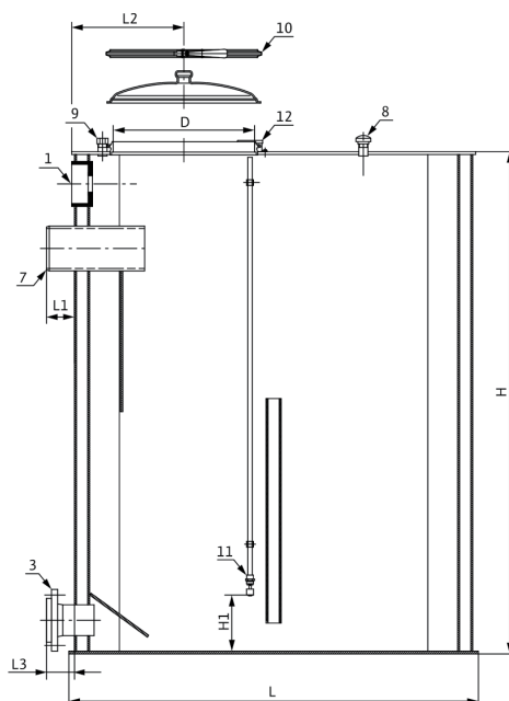
Габаритный чертеж 800 – 1000 л, прямоугольный
