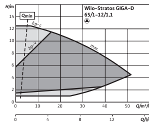
Stratos GIGA-D 65/1-12/1,1
