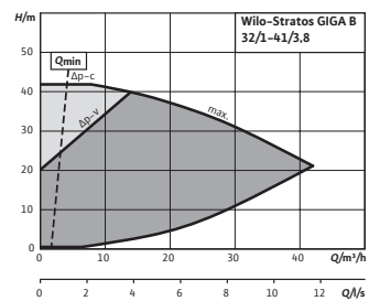
Courbe caractéristique Stratos GIGA B 32/1-41/3,8
