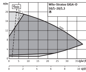
Stratos GIGA-D 50/1-20/1,3
