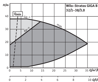
Courbe caractéristique Stratos GIGA B 32/1-38/3,0
