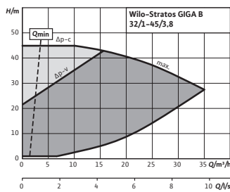
Courbe caractéristique Stratos GIGA B 32/1-45/3,8
