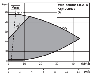
Stratos GIGA-D 50/1-50/4,2
