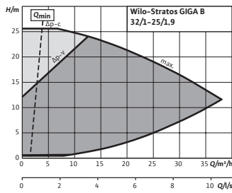
Courbe caractéristique Stratos GIGA B 32/1-25/1,9
