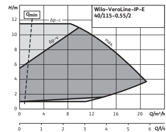
Courbe caractéristique
