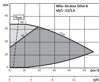
Courbe caractéristique Stratos GIGA B 40/1-33/3,0
