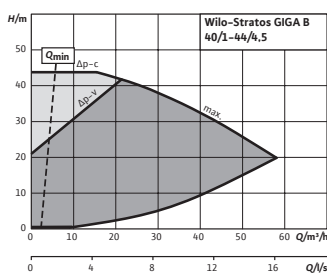
Courbe caractéristique Stratos GIGA B 40/1-44/4,5
