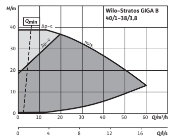
Courbe caractéristique Stratos GIGA B 40/1-38/3,8
