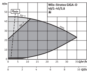
Stratos GIGA-D 40/1-45/3,8
