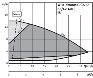
Stratos GIGA-D 50/1-14/0,8
