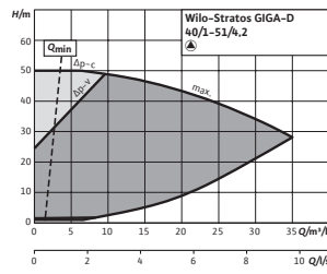
Stratos GIGA-D 40/1-51/4,2
