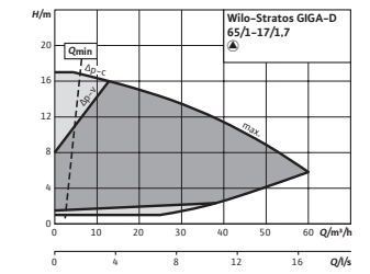
Stratos GIGA-D 65/1-17/1,7
