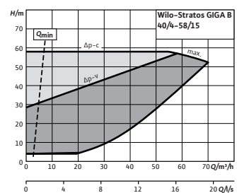
Courbe caractéristique Wilo-Stratos GIGA B 40/4-58/15
