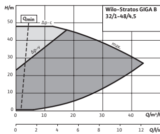
Courbe caractéristique Stratos GIGA B 32/1-48/4,5
