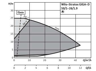
Stratos GIGA-D 50/1-26/1,9
