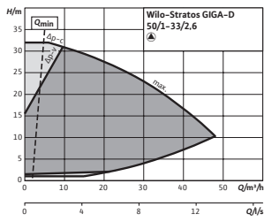
Stratos GIGA-D 50/1-33/2,6
