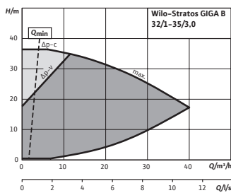
Courbe caractéristique Stratos GIGA B 32/1-35/3,0
