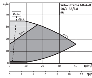
Stratos GIGA-D 50/1-38/2,8
