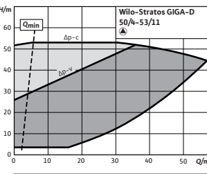
Stratos GIGA-D 50/4-53/11
