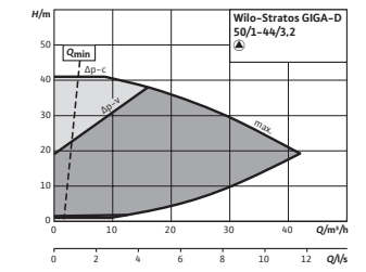
Stratos GIGA-D 50/1-44/3,2
