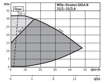
Courbe caractéristique Stratos GIGA B 32/1-32/2,6
