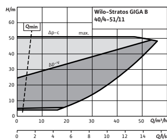
Courbe caractéristique Wilo-Stratos GIGA B 40/4-51/11
