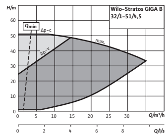
Courbe caractéristique Stratos GIGA B 32/1-51/4,5
