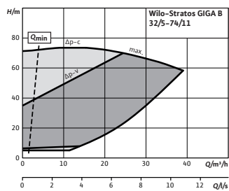
Courbe caractéristique Wilo-Stratos GIGA B 32/5-74/11
