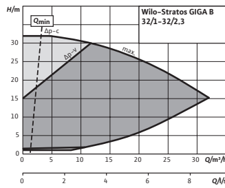
Courbe caractéristique Stratos GIGA B 32/1-32/2,3
