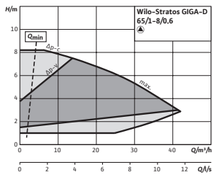
Stratos GIGA-D 65/1-8/0,6
