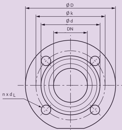
Flange PN 6 for 3 NPS
