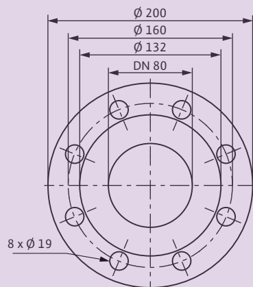
Flange PN 10 for 3 NPS
