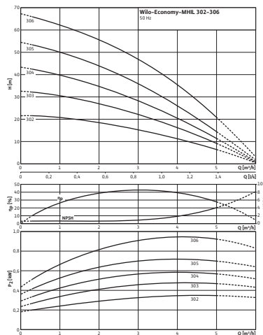
Charakteristiky dle ISO 9906, třída 2
