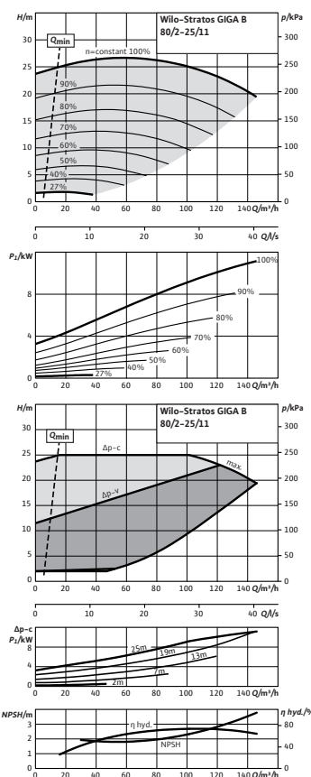
Charakteristika čerpadla
