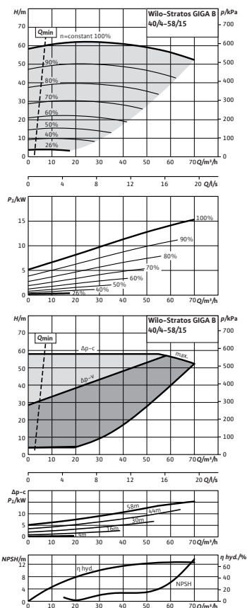
Charakteristika čerpadla
