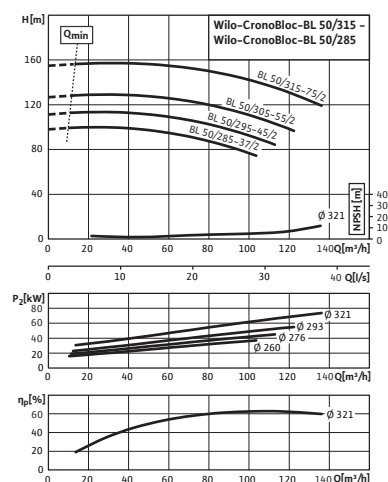
Charakteristika čerpadla
