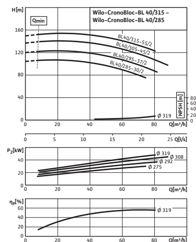
Charakteristika čerpadla
