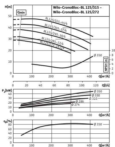
Charakteristika čerpadla
