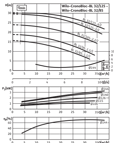
Charakteristika čerpadla
