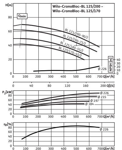
Charakteristika čerpadla
