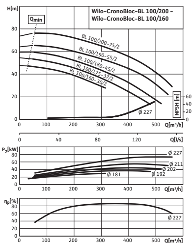
Charakteristika čerpadla
