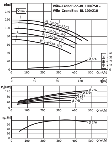
Charakteristika čerpadla
