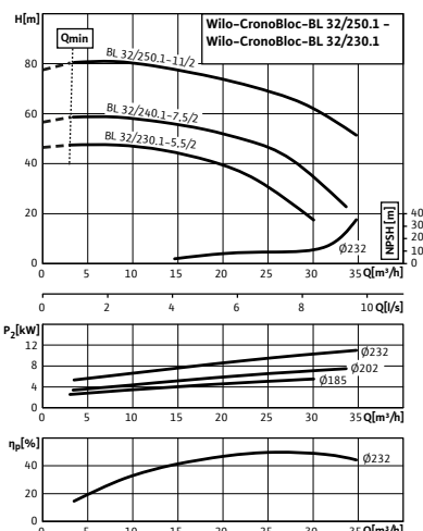
Charakteristika čerpadla
