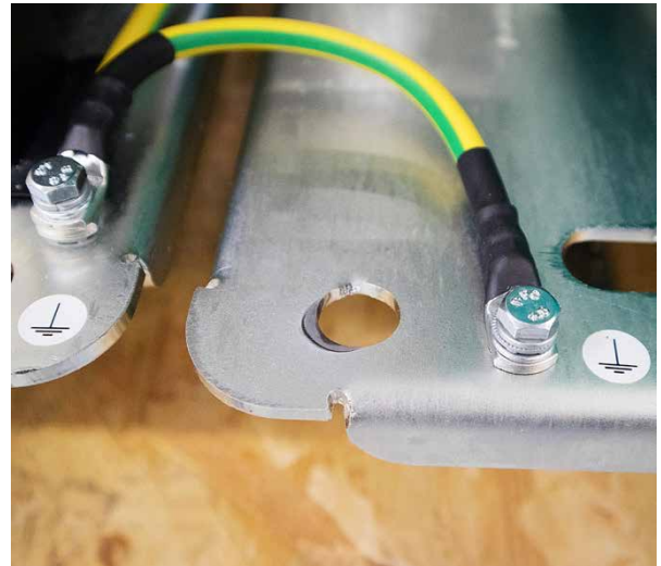
Montierte Erdung.
