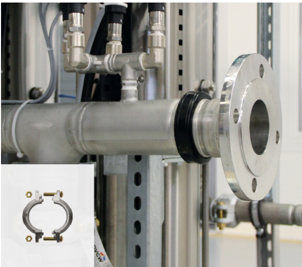
3. Flansch einfügen.
