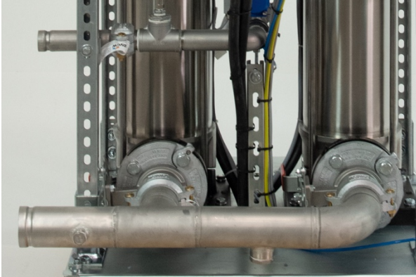
Rohranschluss Saugseite.
