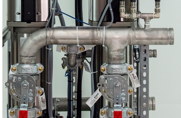
Rohranschluss Betriebswasser.
