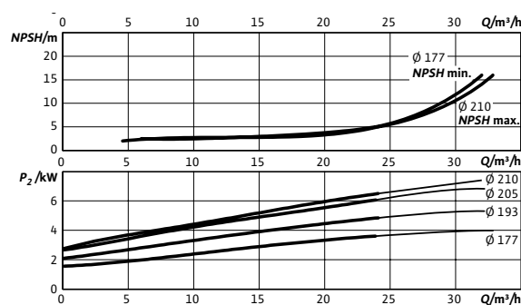
Rys. 2 Wykres przedstawiający wznoszącą charakterystykę mocy (P2)
