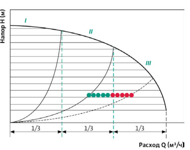
Рабочая точка перемещается в область II (средняя треть).
