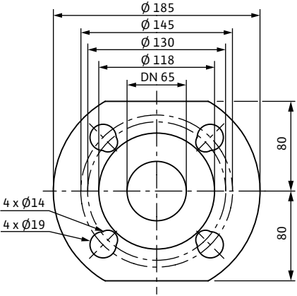
Пример комбинированного фланца PN 6/10 для DN 65
