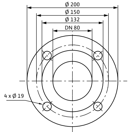
Фланец PN 6 для DN 80
