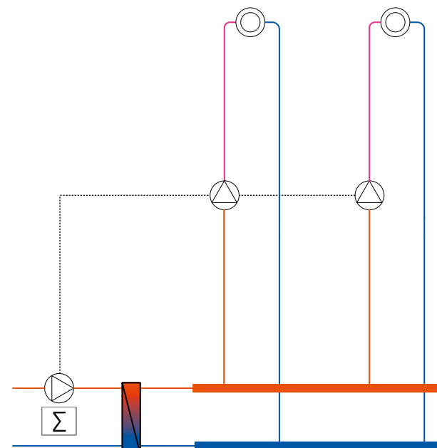
Multi-Flow Adaptation питающего насоса перед теплообменником со вторичными насосами в линии без смесителя
