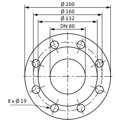
Фланец PN 10 для DN 80
