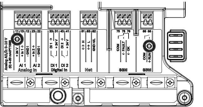
Клеммный отсек Stratos MAXO
