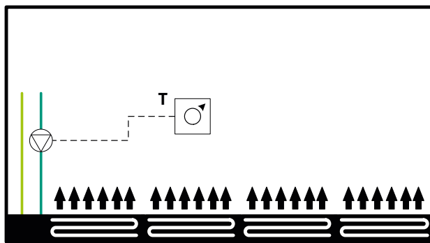
Регулирование температуры в помещении при использовании охлаждения пола в контуре потребителей
