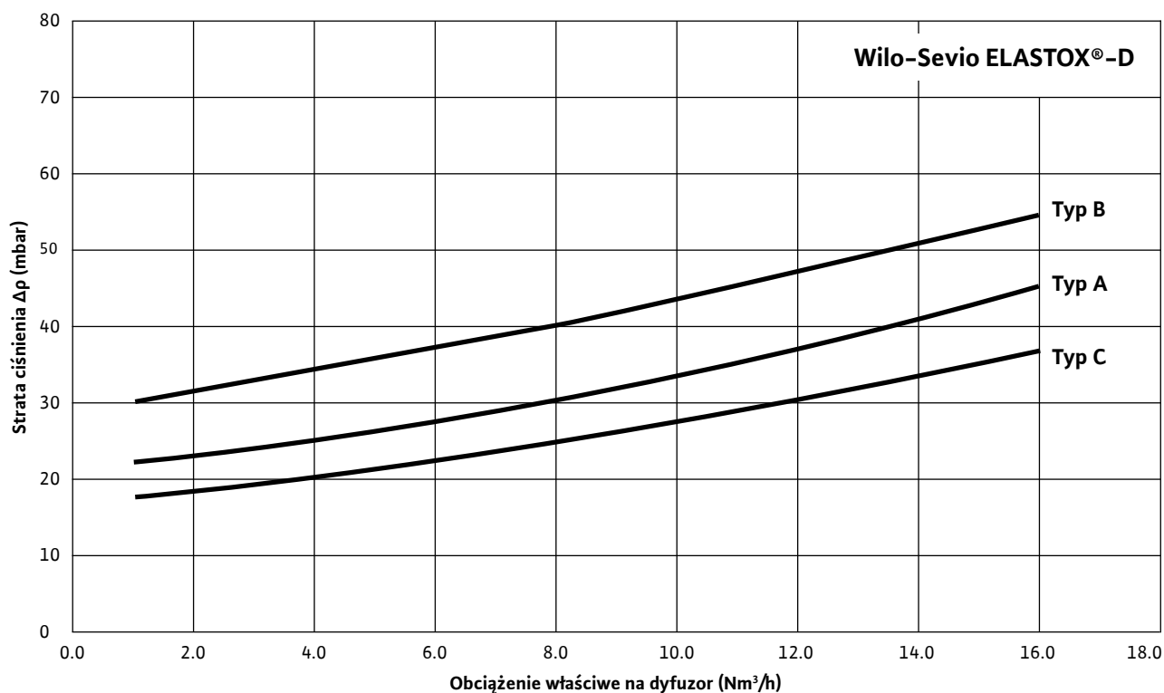
Wykres pracy dyfuzora dyskowego Wilo-Sevio ELASTOX®-D
