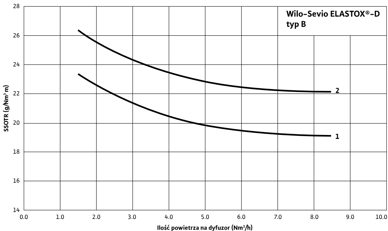
Wykres pracy dyfuzora dyskowego Wilo-Sevio ELASTOX®-D (typ B)
