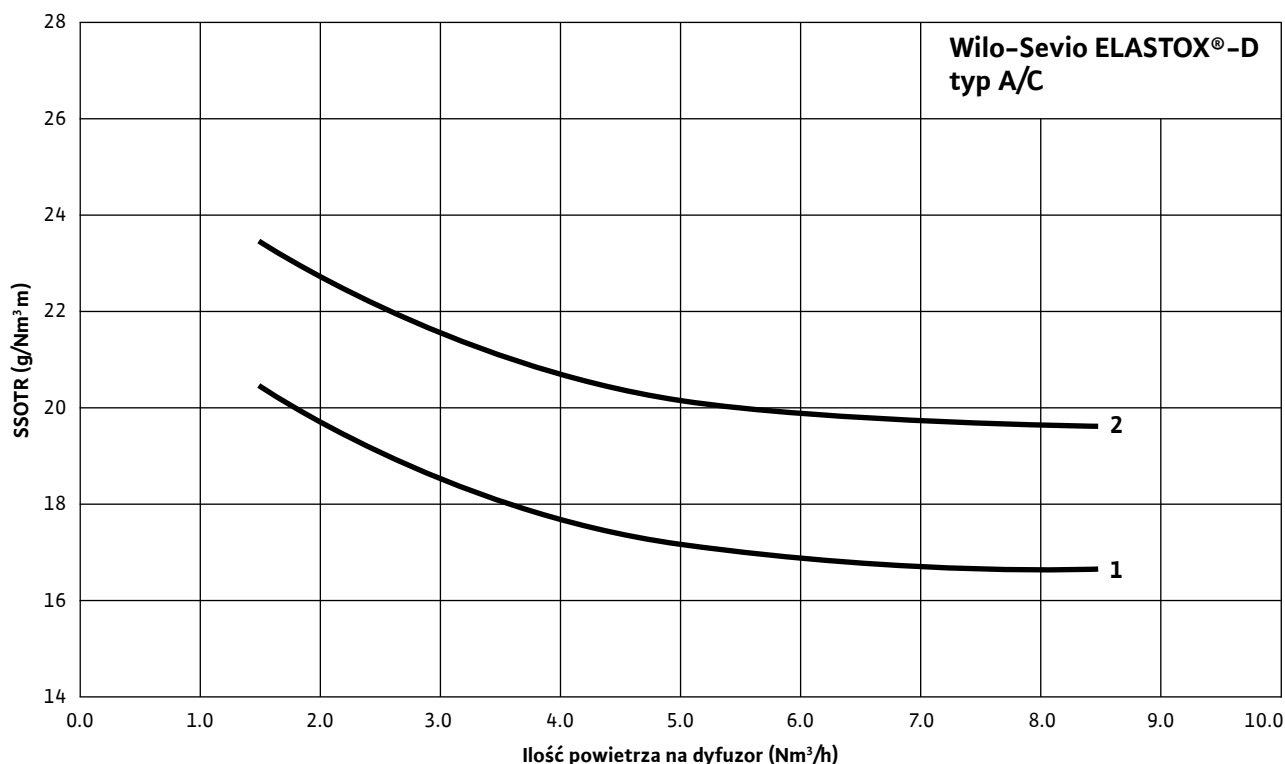
Wykres pracy dyfuzora dyskowego Wilo-Sevio ELASTOX®-D (typ A/C)
