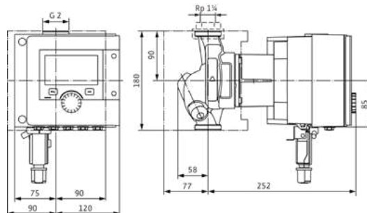
Wilo-Stratos MAXO 30...
