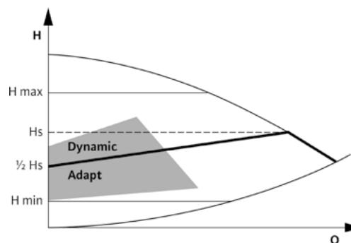
Способ регулирования Др-ν с Dynamic Adapt
