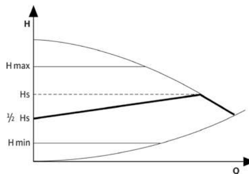
Способ регулирования Др-ν
