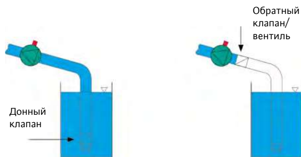
Монтаж с использованием донного клапана и обратного клапана
