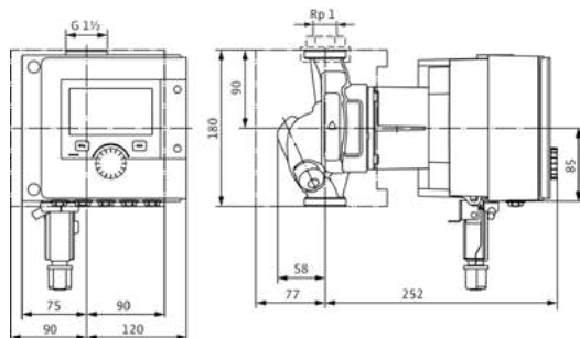
Wilo-Stratos MAXO 25...
